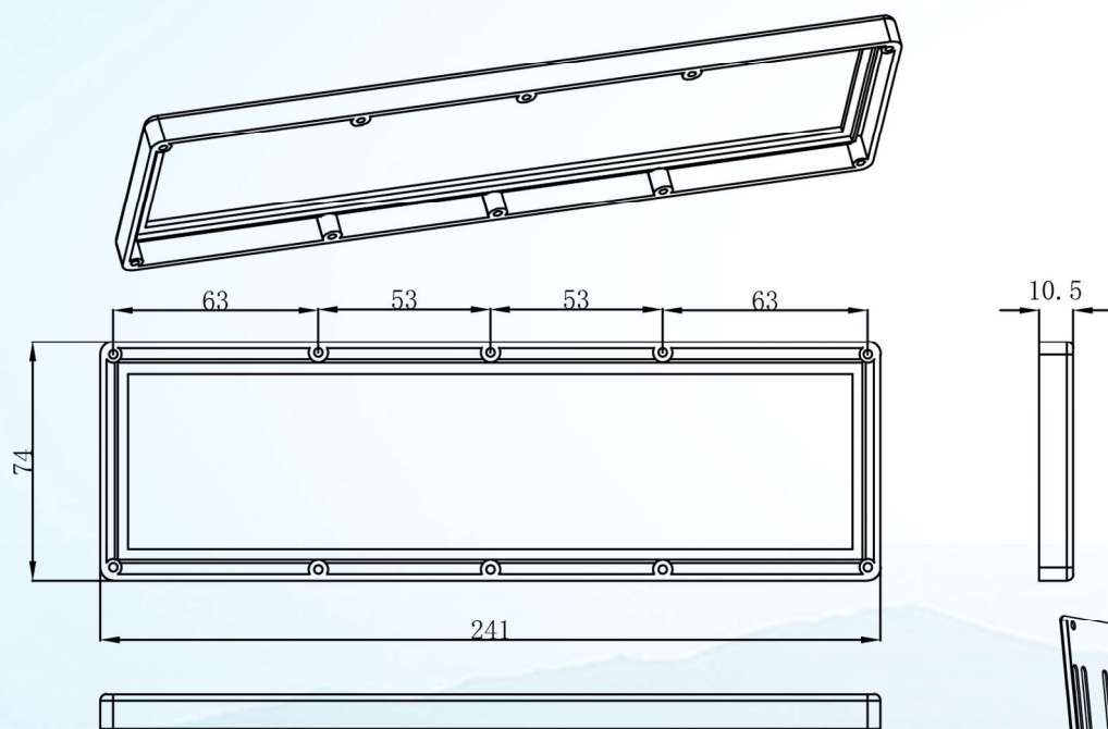
压铸铝面框
