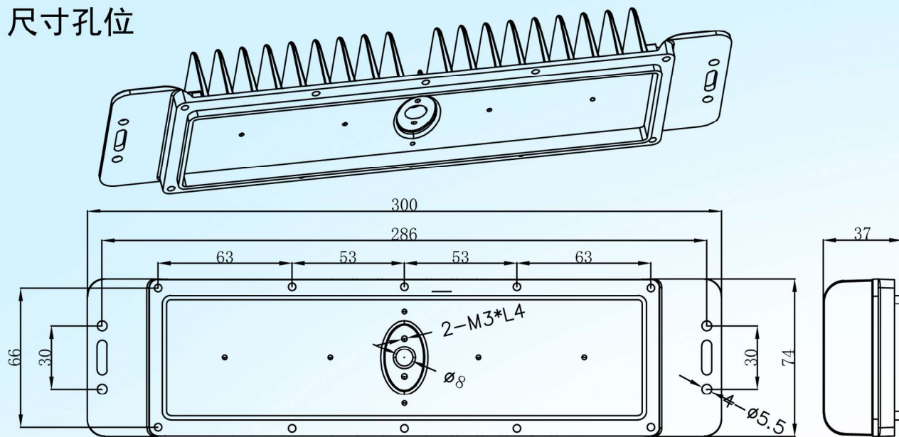
压铸铝灯体
