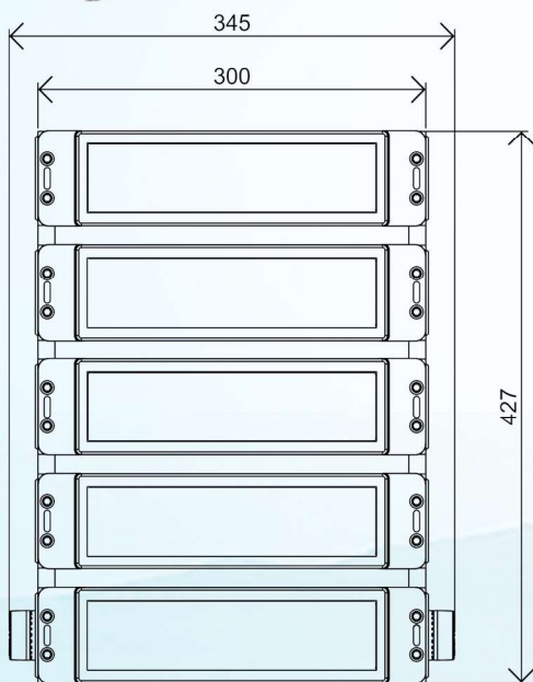
主视图
