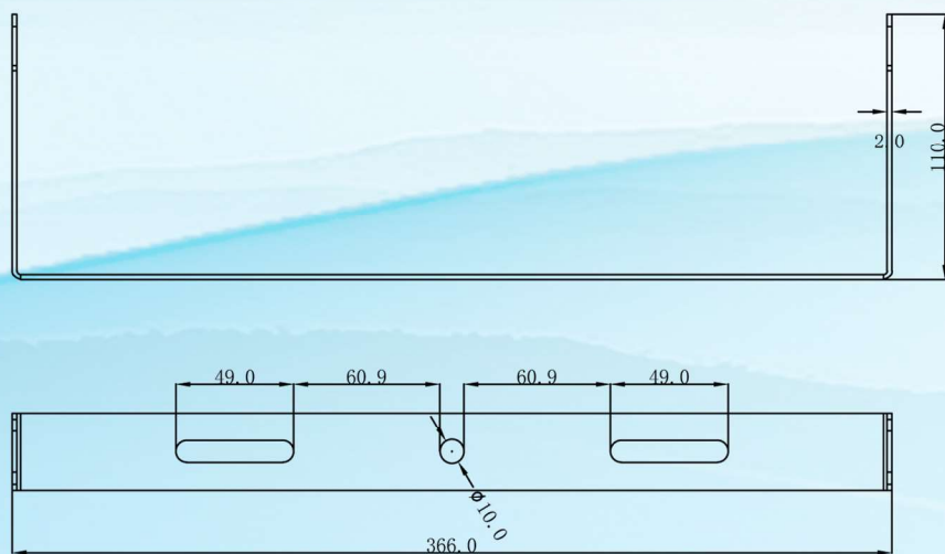
支架孔位
